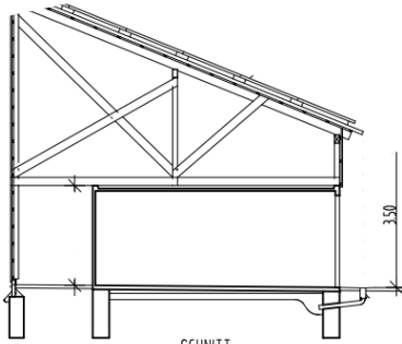
Schnitt WoMo-Garage
